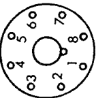
Mazda Octal (M08)
