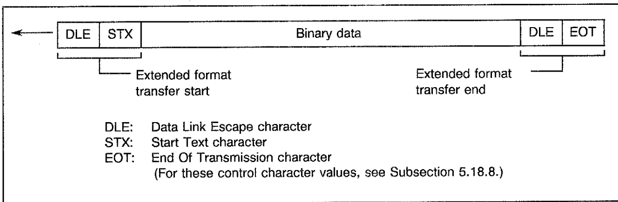
【 Extended Format 】
