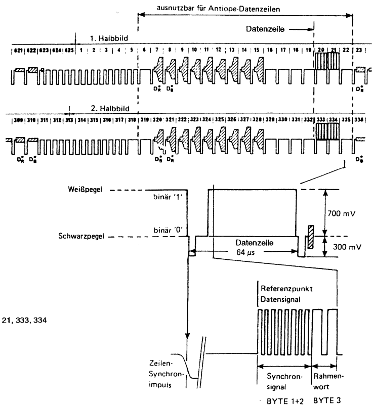
Fig. 3 Lage und Pegel von Antiope-Datenzeilen
