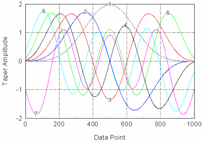
Figure 6.4.3 Slepian SPSS Taper Functions
