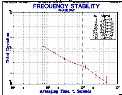
Théo1
