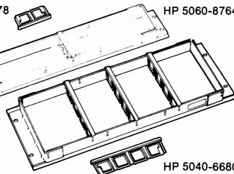
HP 5060-8764
