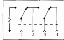
HP 8763 FIG. 2
