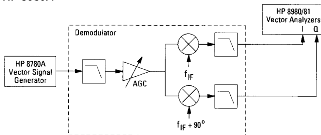
HP 8980A
