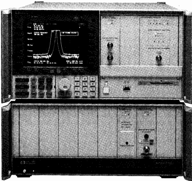
HP 71100C
