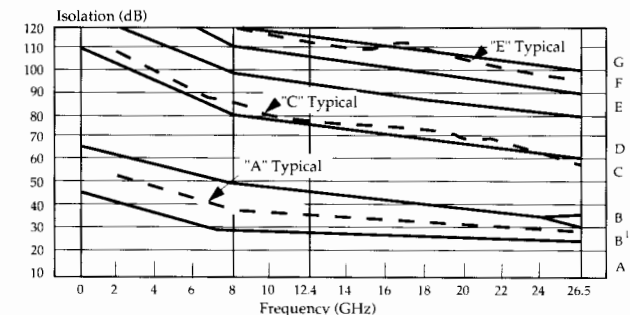
HP 8764 FIG. 3
