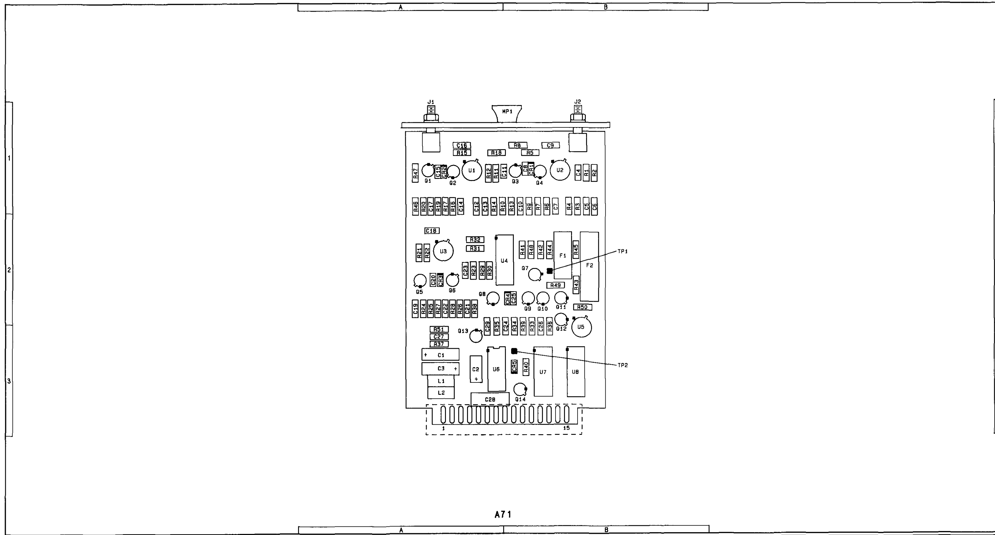
A71 Component Locator
