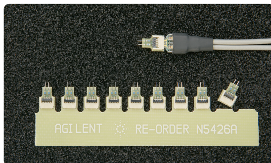
Figure 8. New InfiniiMax ZIF probe head (N5425A) and ZIF tips (N5426A) for your DDR2 probing solution.
