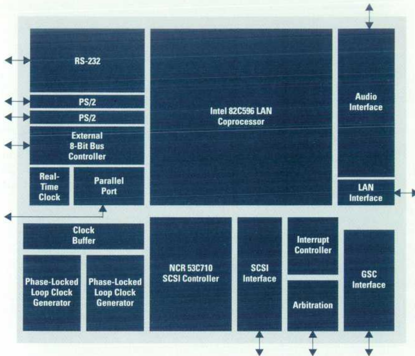
Fig. 2. LASI floorplan.
