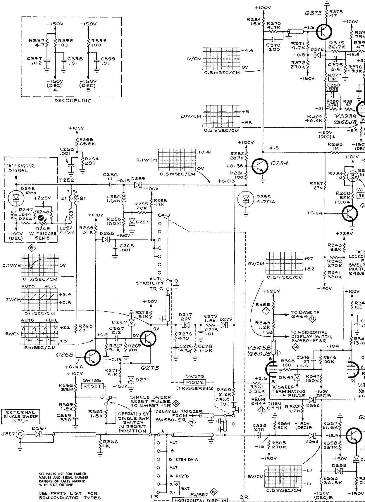
† TYPE 547 OSCILLOSCOPE
