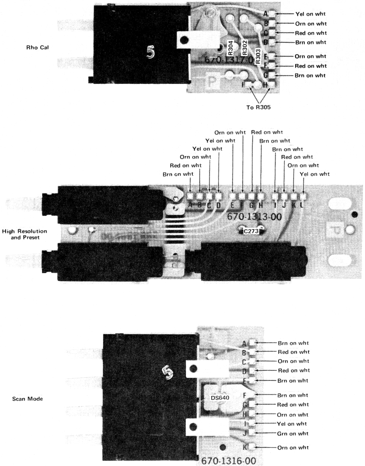
Fig. 7-7. Assemblies A-7, A-8, and A-9.
