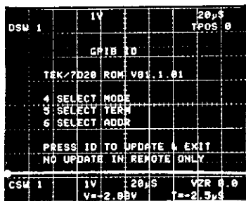
Figure 2-67. ID MENU.
