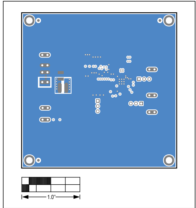
MAX17504EVKITBE# PCB Layout—Bottom Layer
