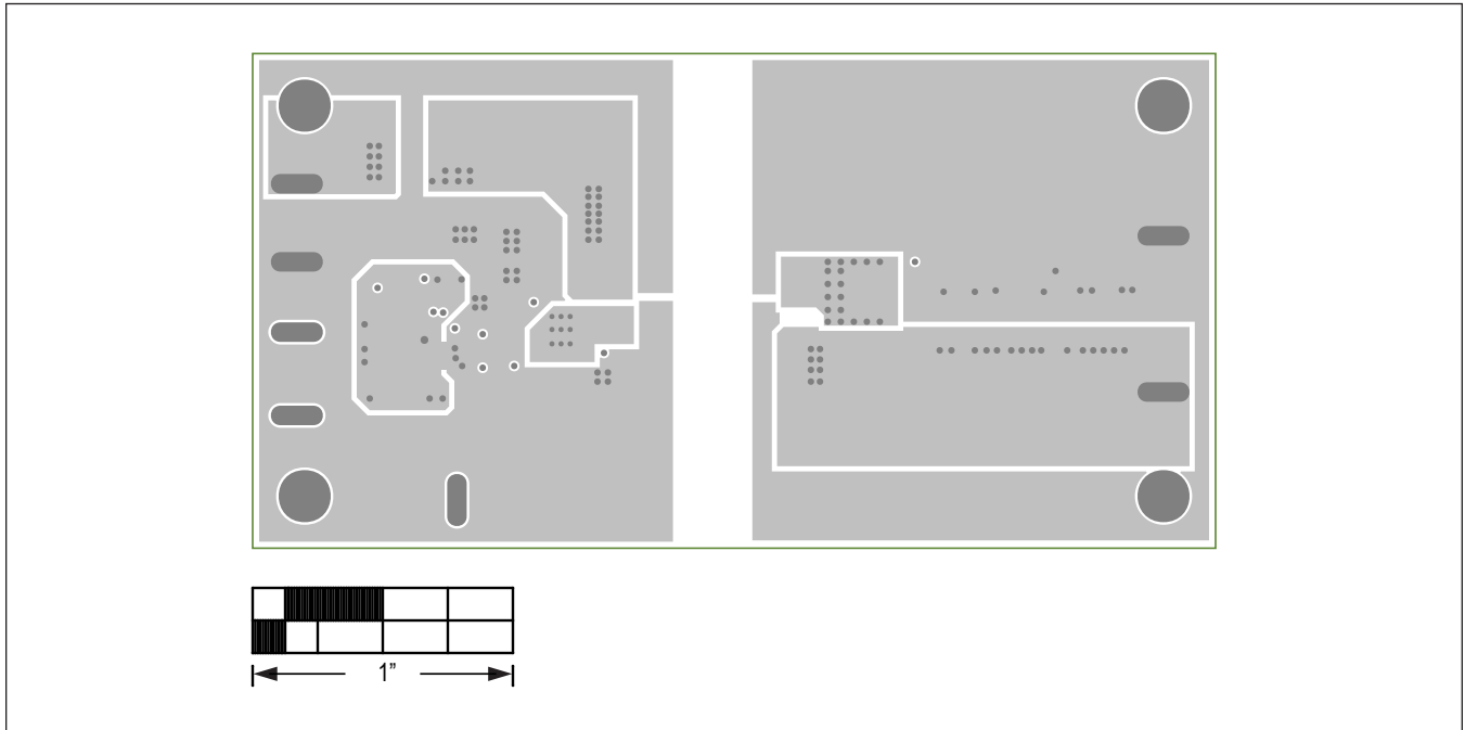
INNERLAYER2
