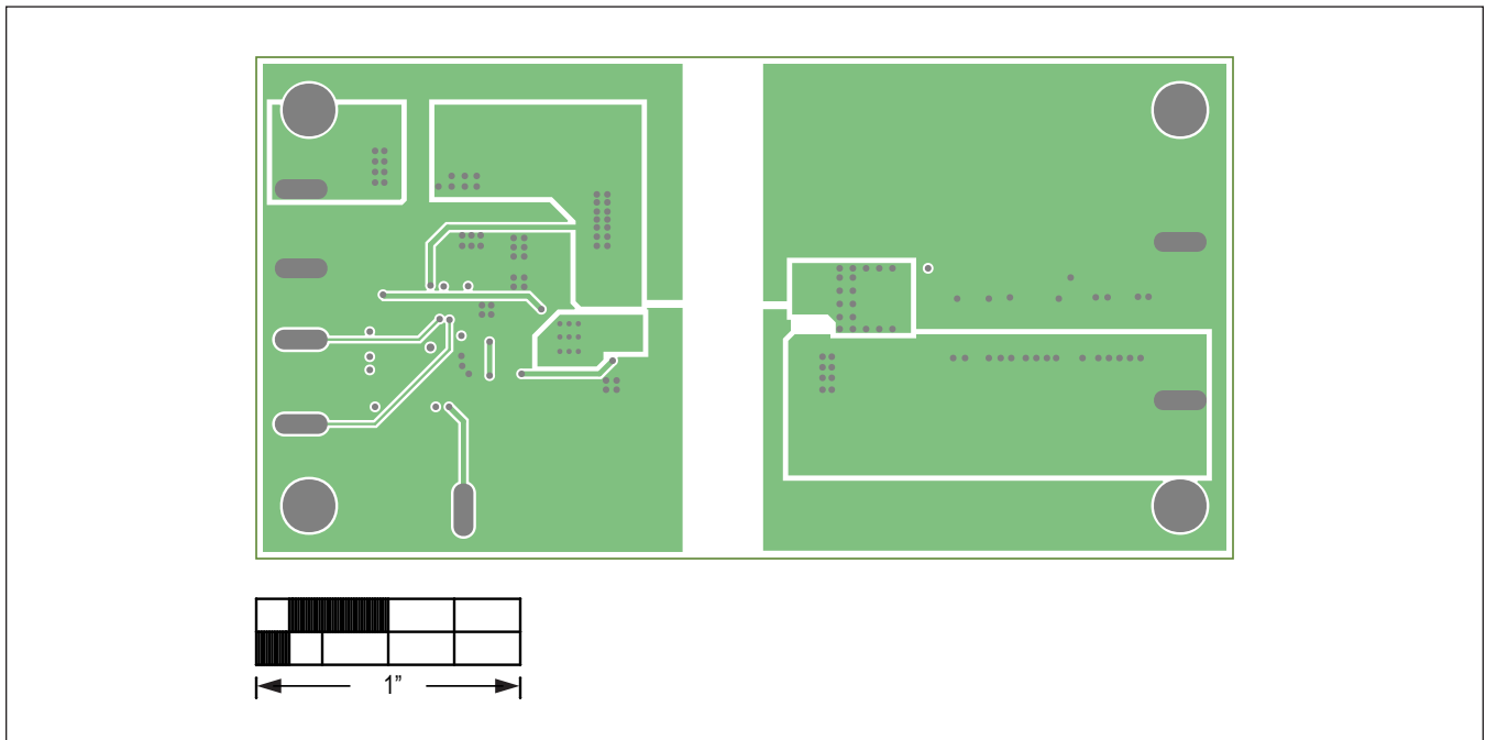
INNERLAYER3
