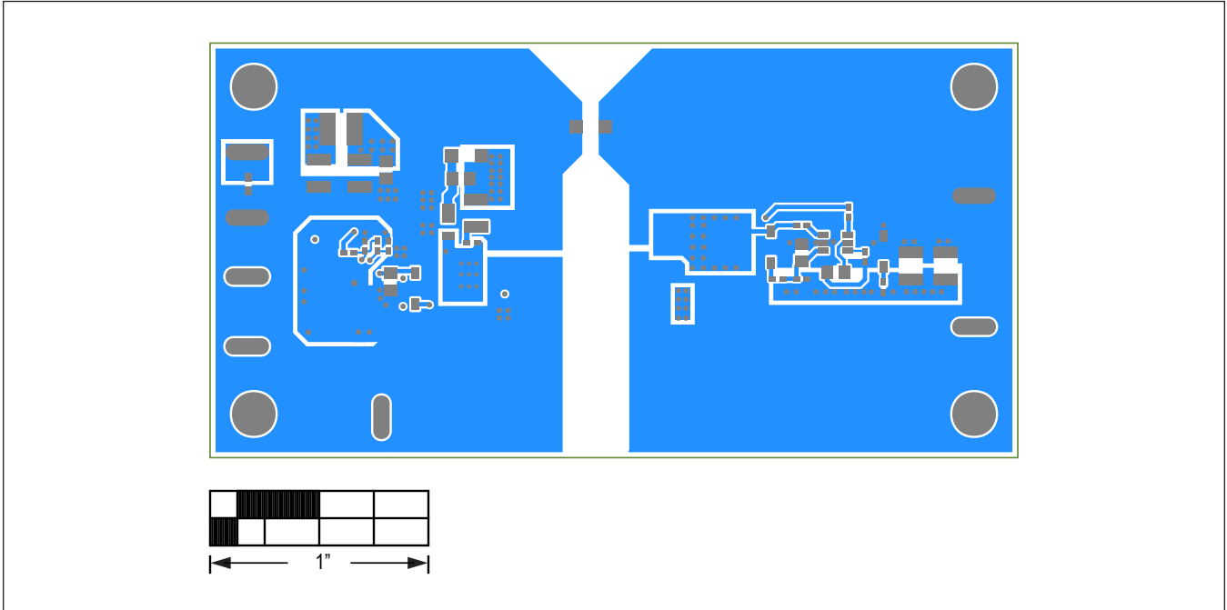
Bottom
