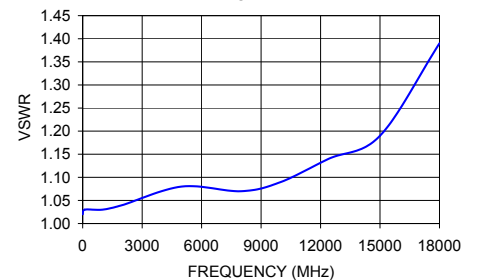
BW-S10W2+ VSWR
