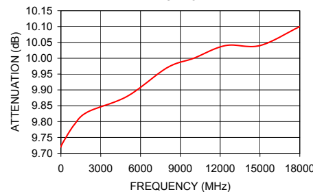
BW-S10W2+ ATTENUATION
