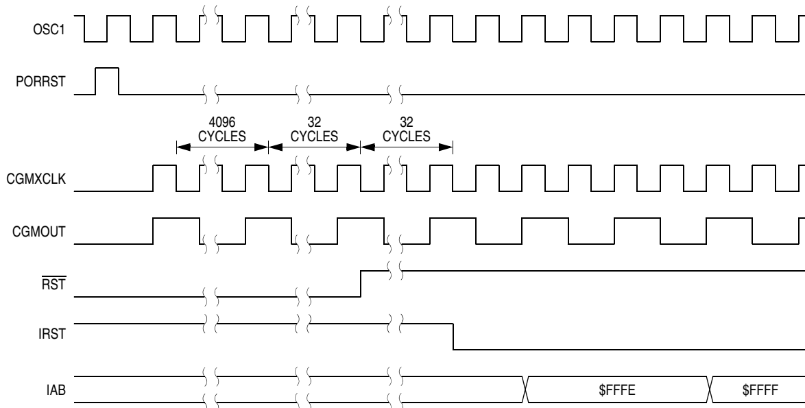
Figure 15-8. POR Recovery
