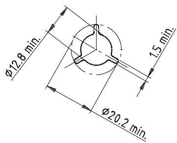
Reel hub 2:1
