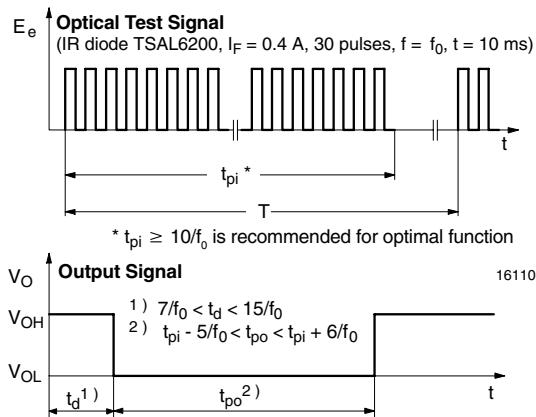
Fig. 1 - Output Function
