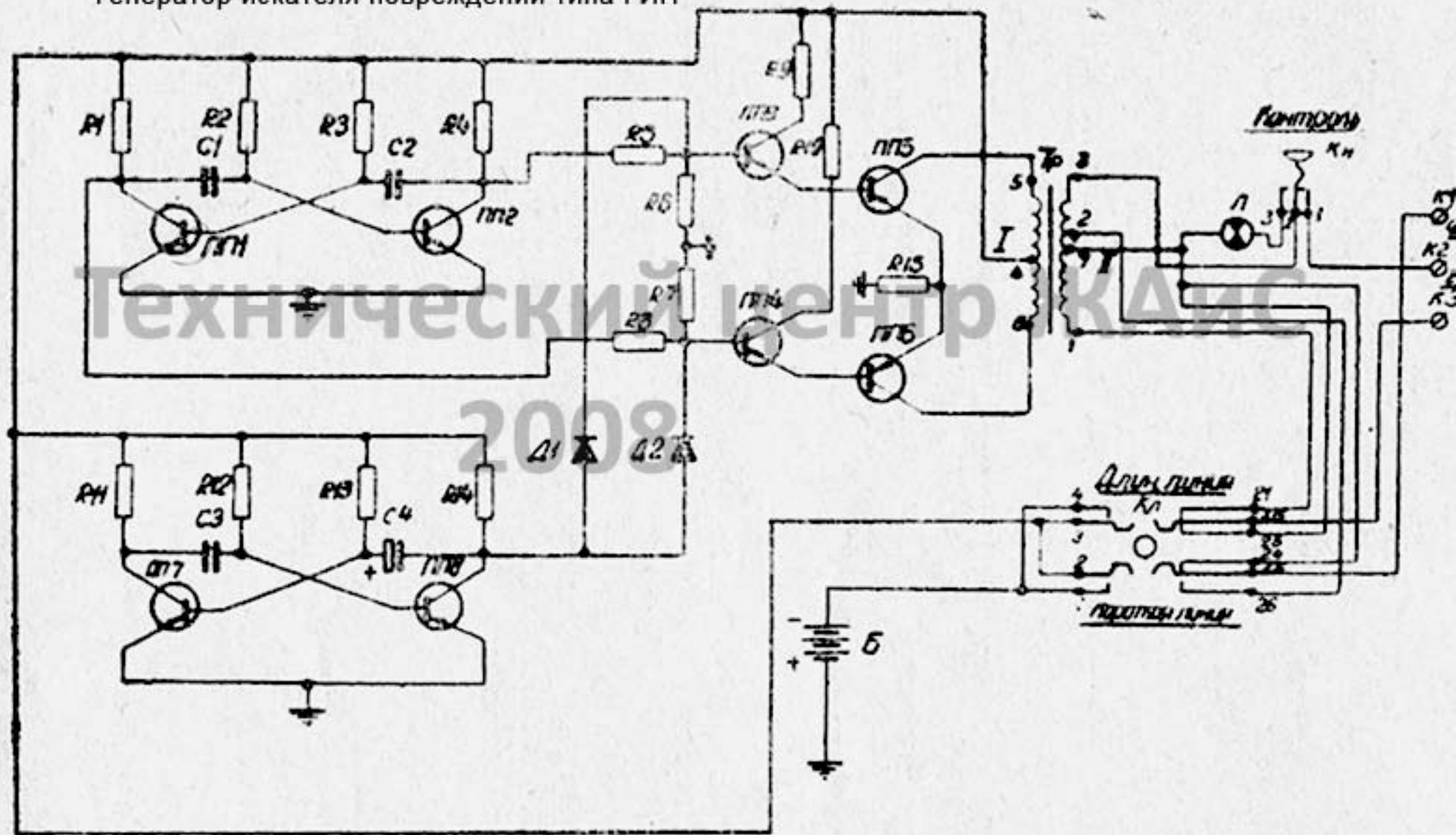
Генератор искателя повреждений типа ГИП
