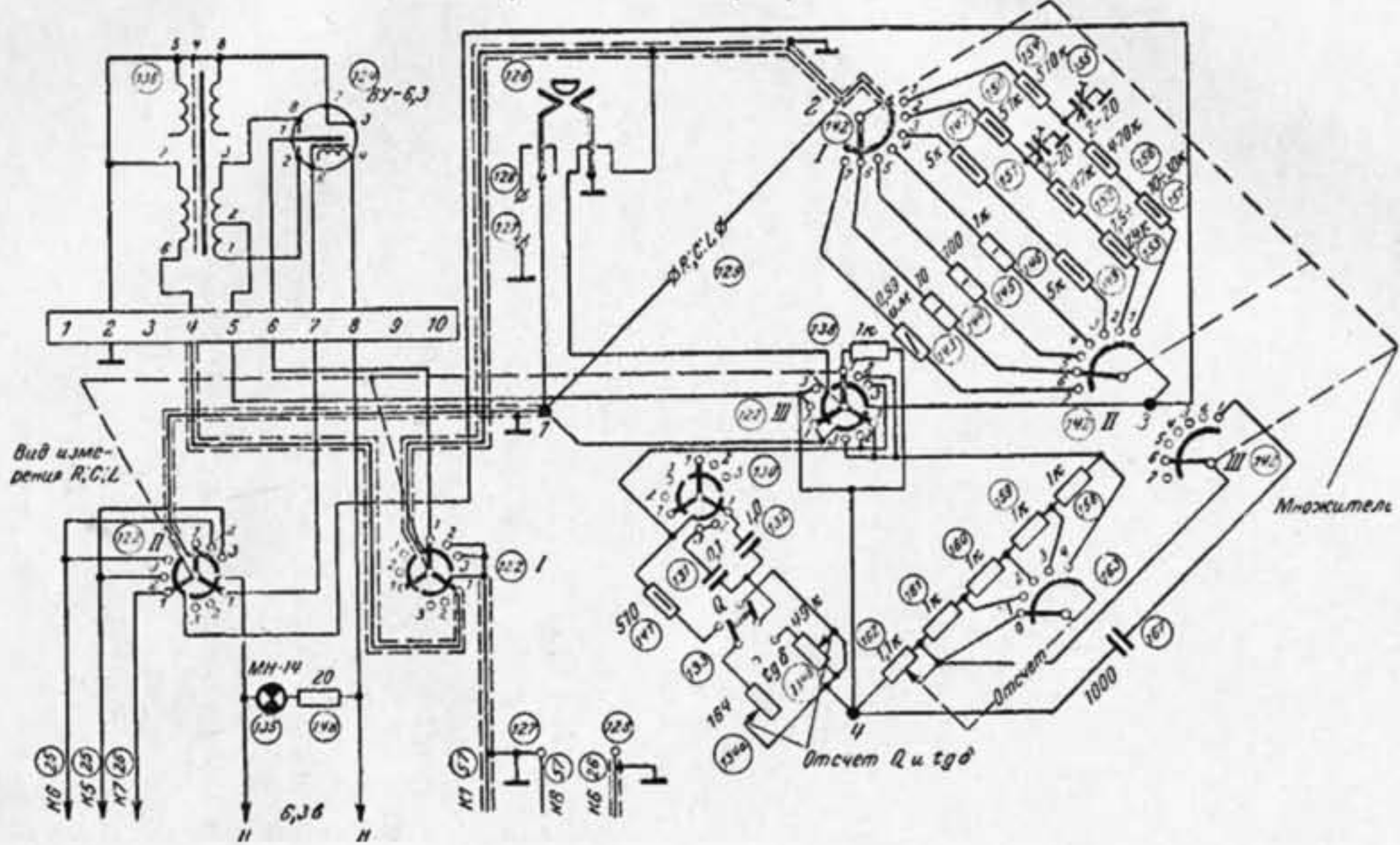
Схема измерительного моста прибора Е12-2.
