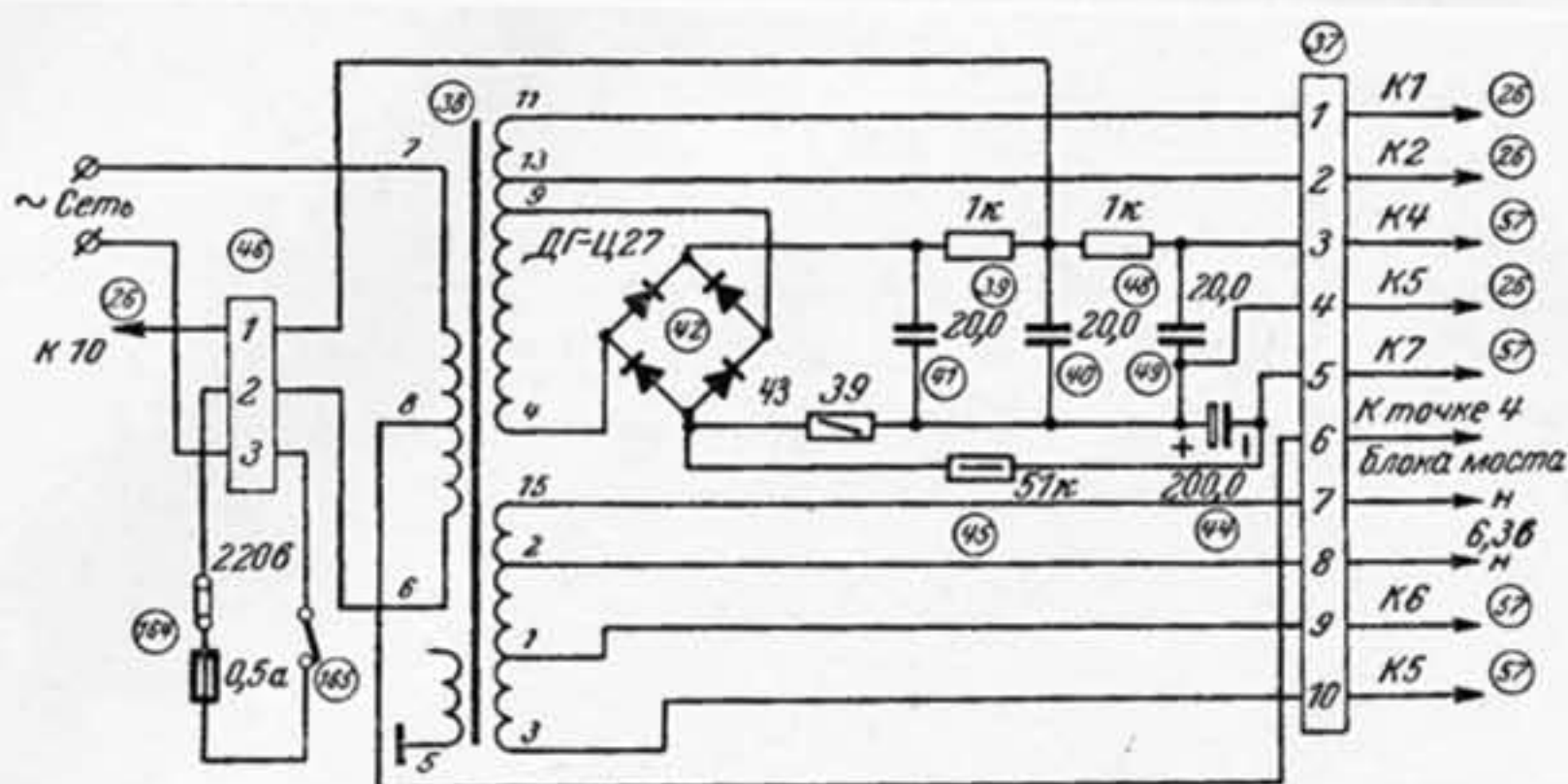
Схема блока выпрямителя прибора Е12-2.
