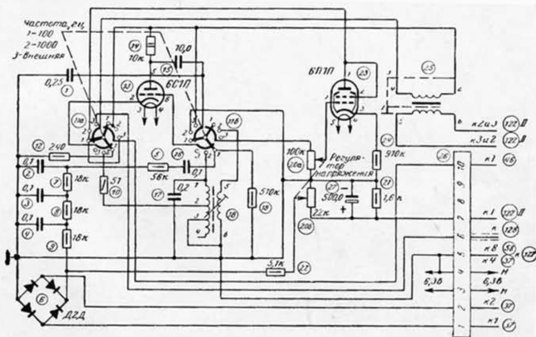
Схема блока генератора прибора Е12-2.
