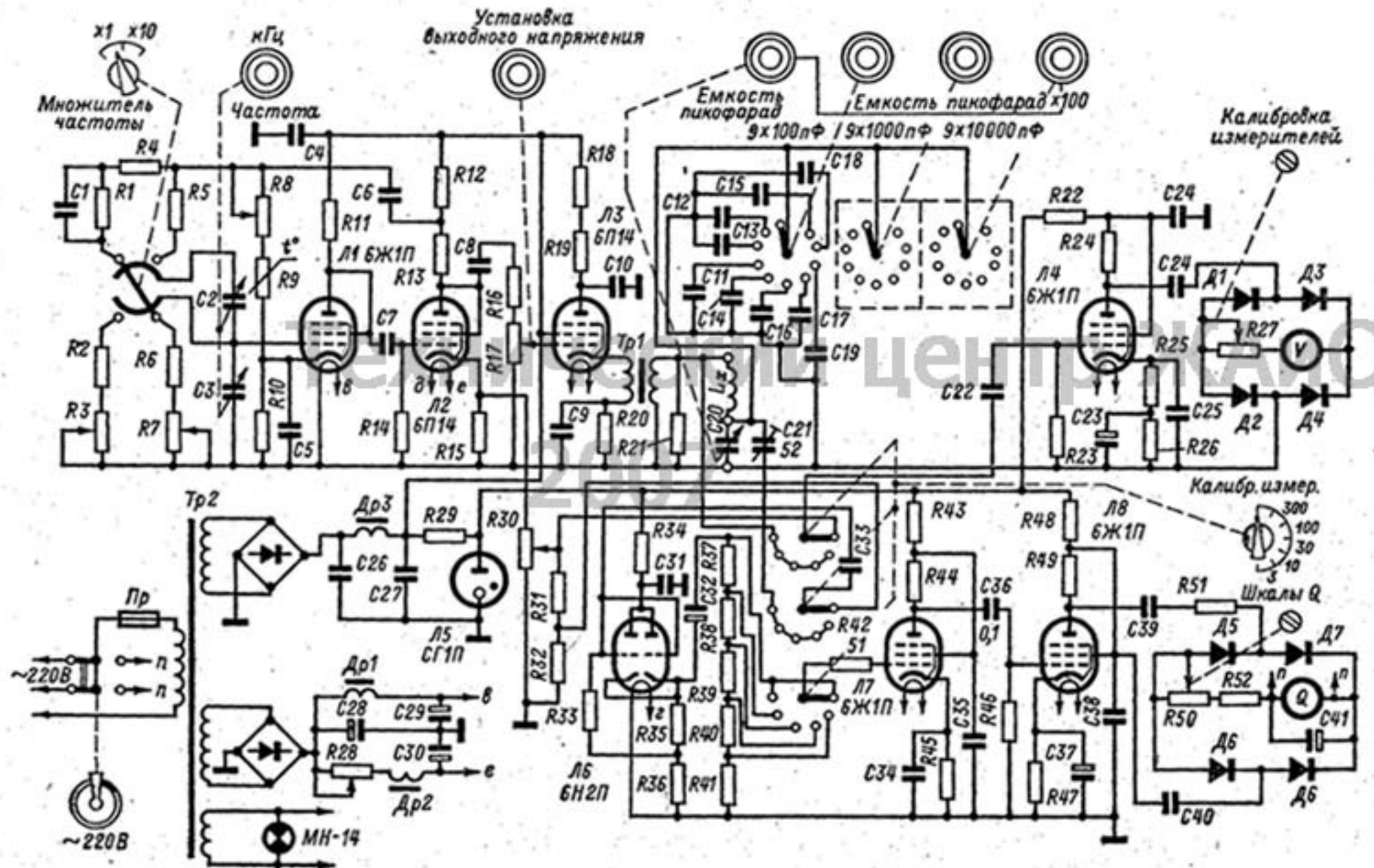
Электрическая принципиальная схема измерителя добротности низкочастотного Е4-3.
