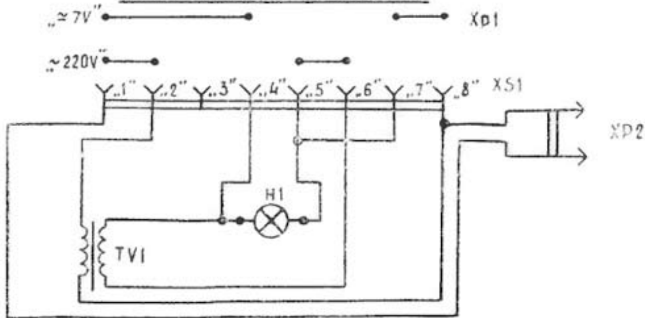
Схема питания освещения
