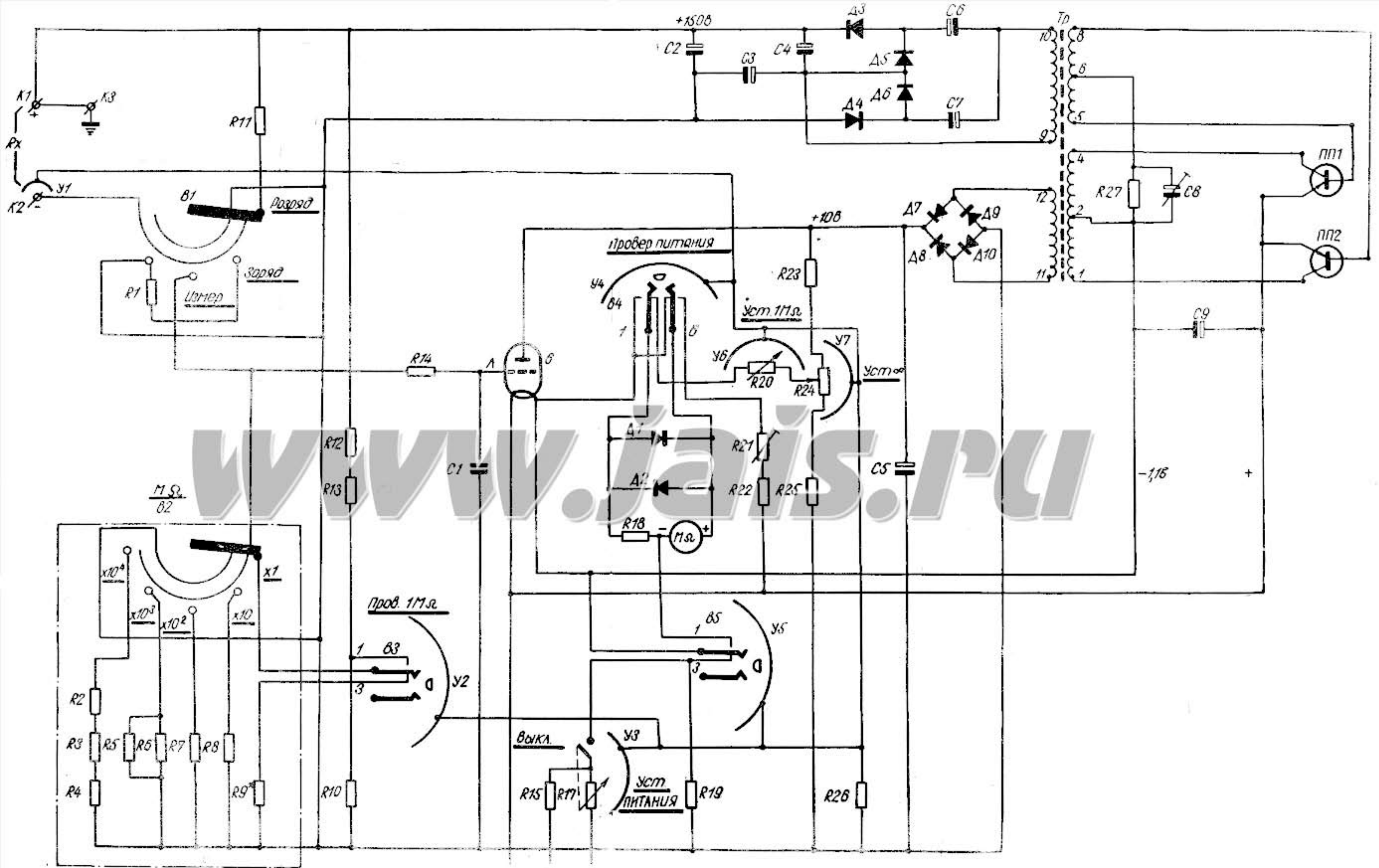
Рис. 6. Мегаомметр МEG-9. Схема принципиальная электрическая — РХ2 722 005 СхЭ
