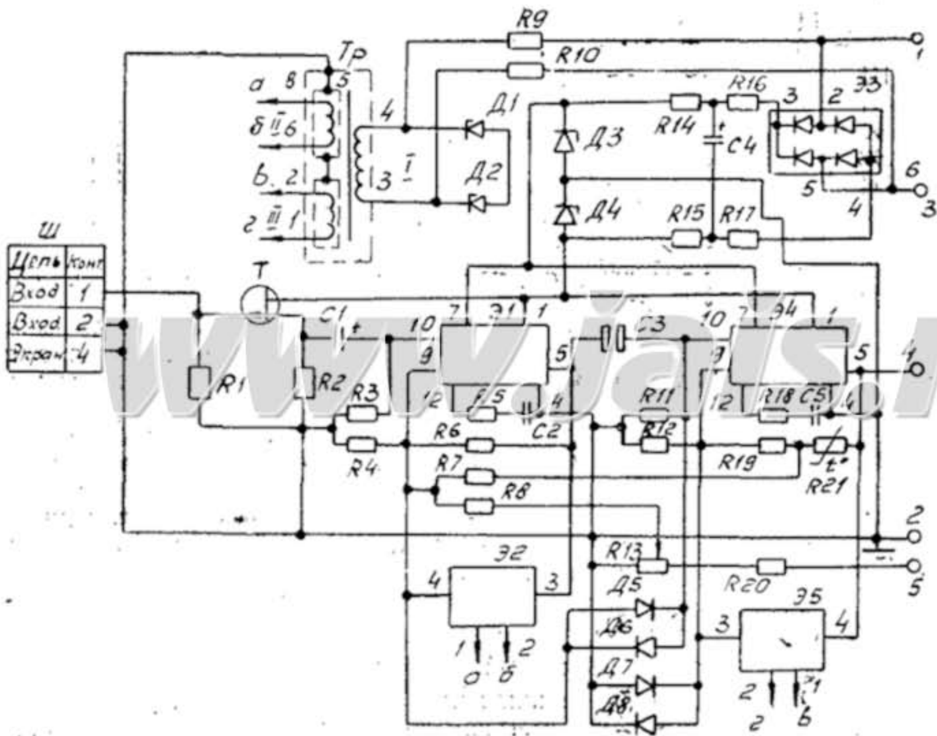
Усилитель предварительный
