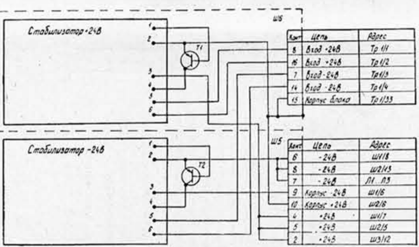
Схема электрическая принципиальная блока стабилизатора
